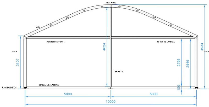
ALZADO FRONTAL
