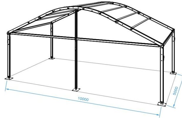
REPRESENTACIÓN 3D
