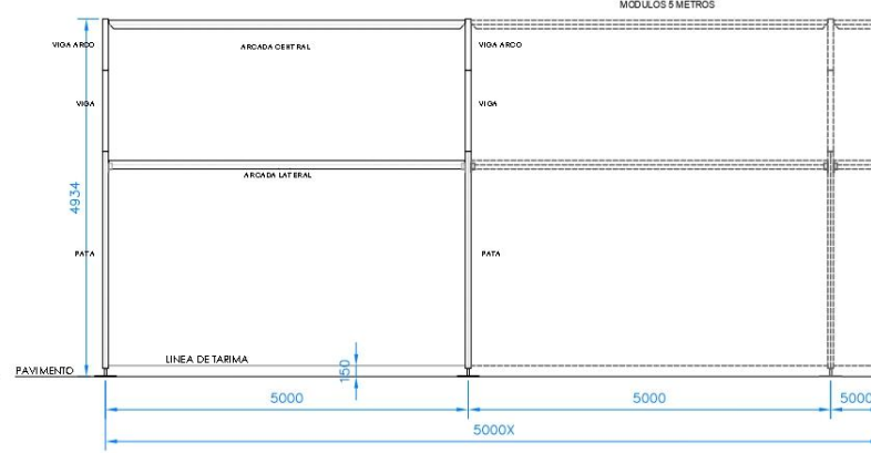
ALZADO LATERAL
