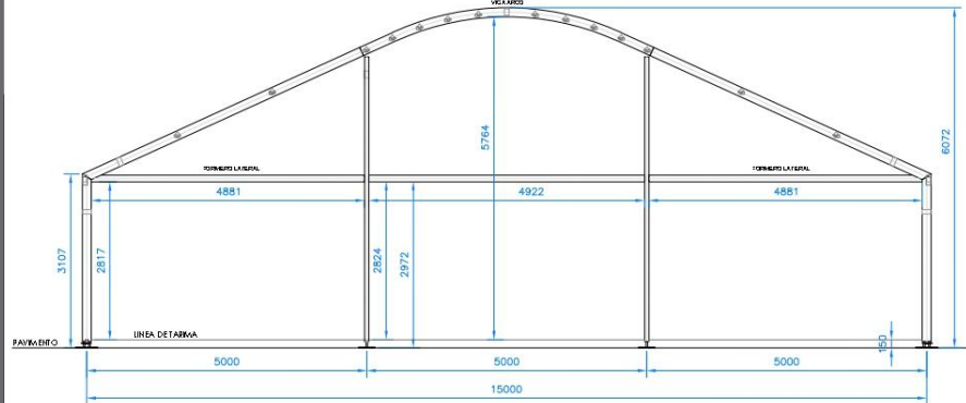
ALZADO FRONTAL
