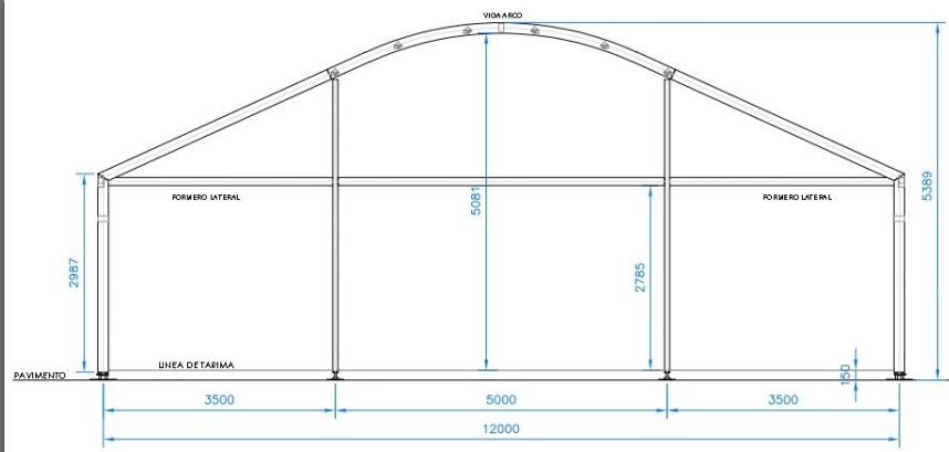
ALZADO FRONTAL
