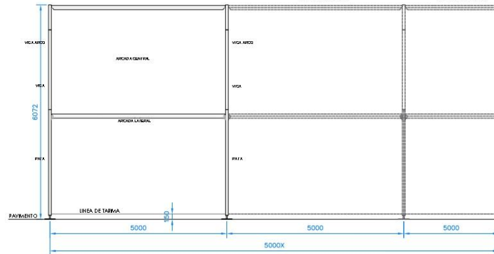
ALZADO LATERAL
