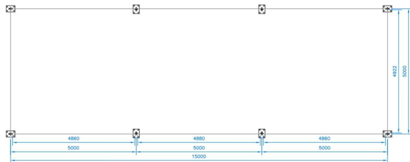
PLANTA
