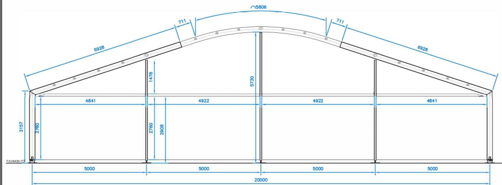
ALZADO FRONTAL
