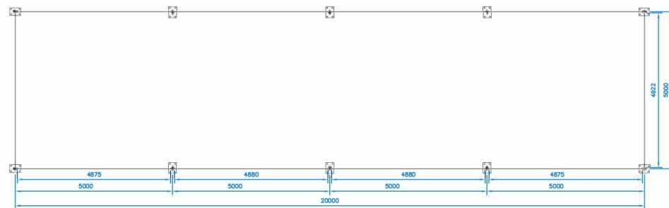
PLANTA
